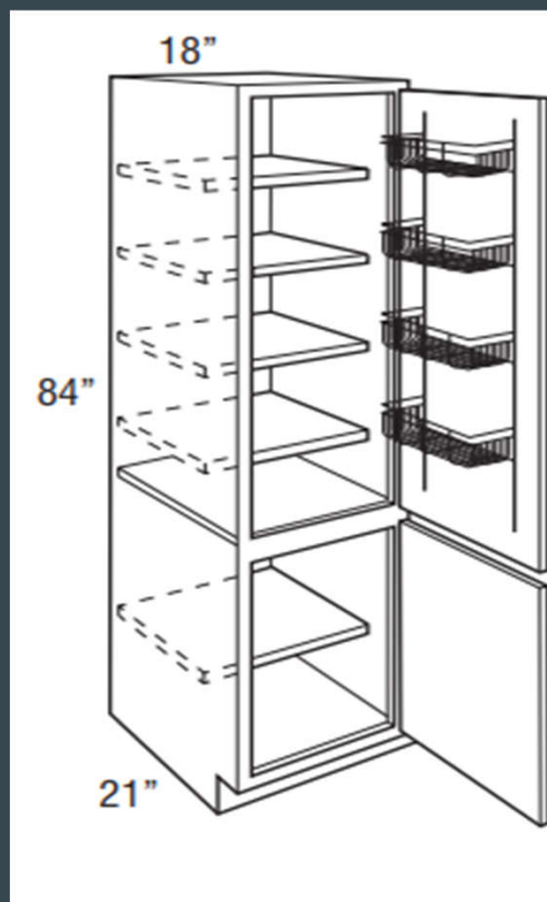
LINEN CLOSET
